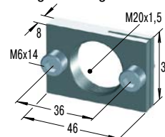
RF20 Flangia rettangolare
